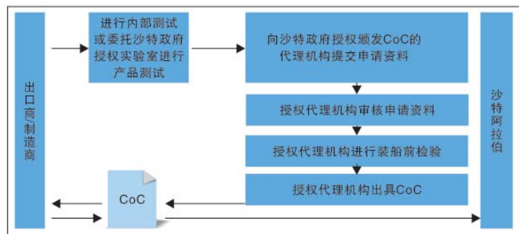
图2 出运前符合性验证流程
