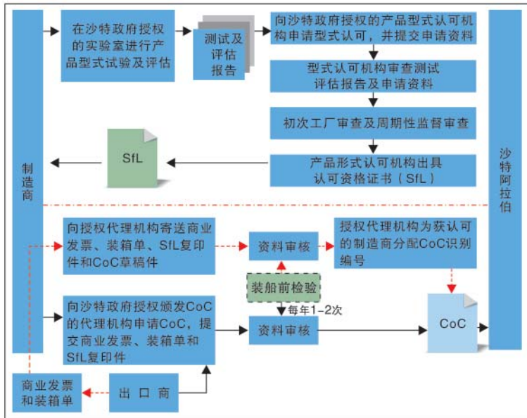
图4 产品型式认可流程
